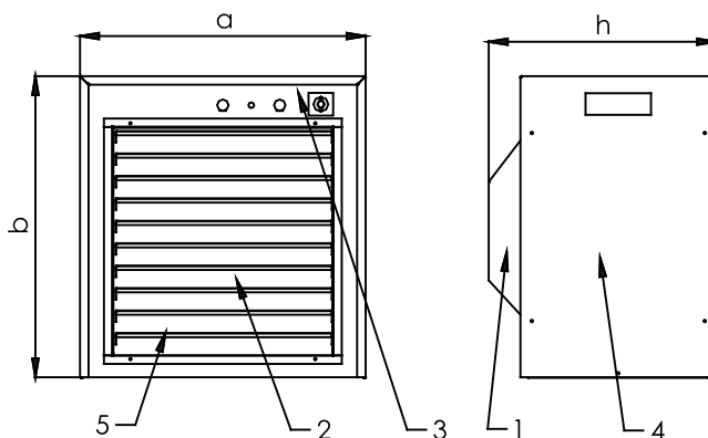
Rys. 1 Budowa aparatu
